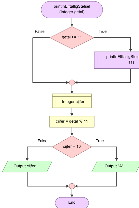
Figuur 7.8: Een recursief algoritme om een getal om te zetten naar het elftalig stelsel.
