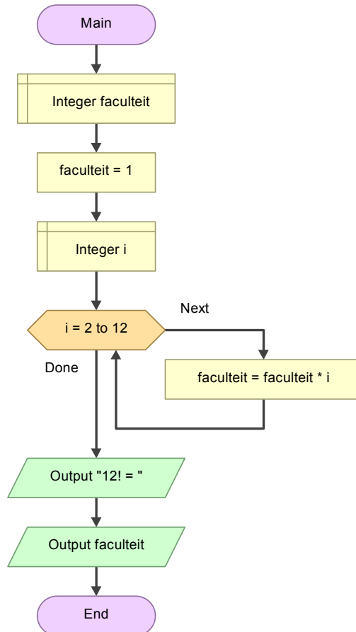
Figuur 4.3: De flowchart van het programma uit listing 4.3 .
