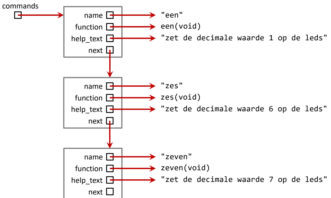
Figuur 2: Een mogelijke datastructuur om de commando's in op te slaan.
