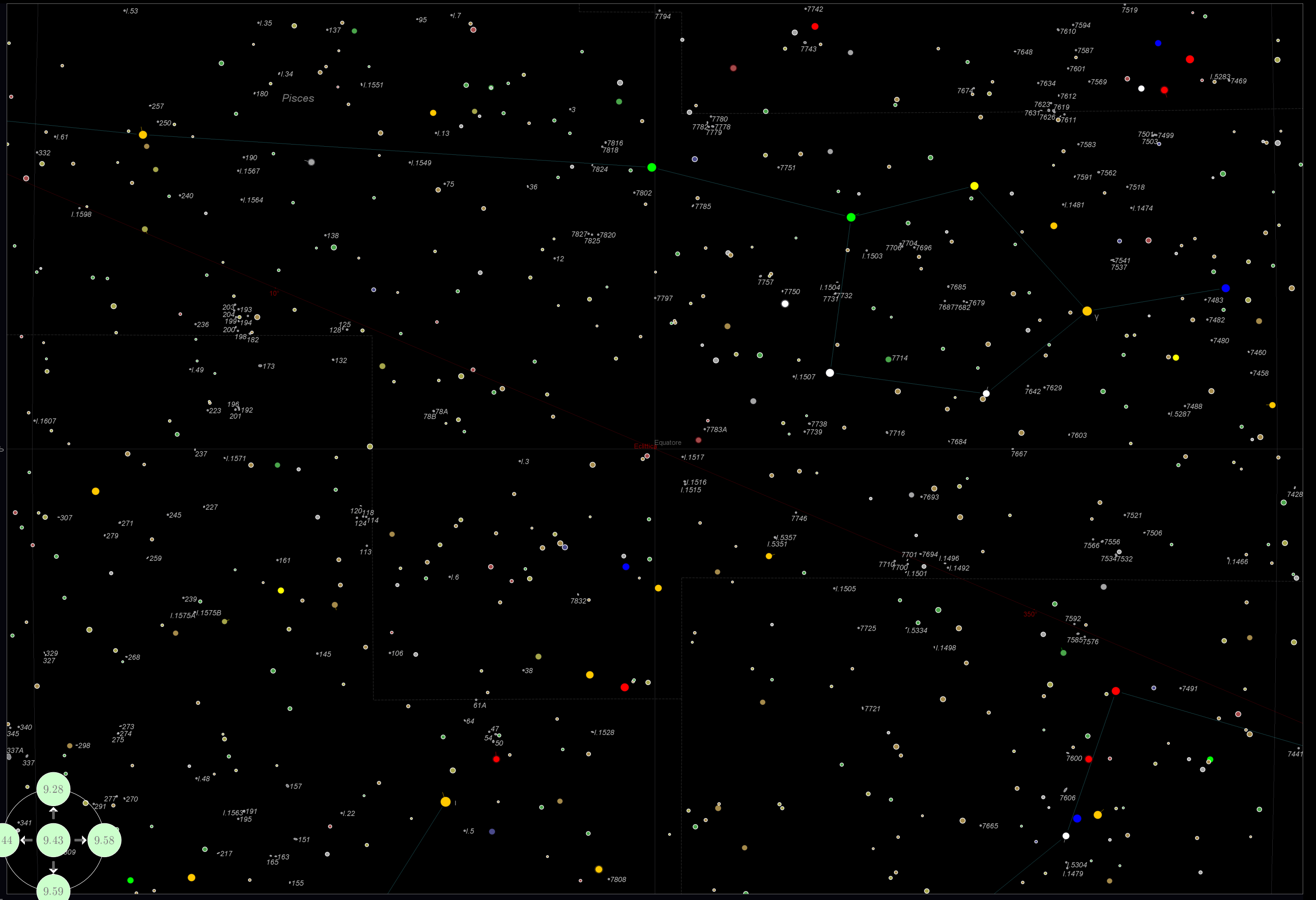
9.43 Mappa 43 25° attorno 0.0h, 0.0° (Pisces)
