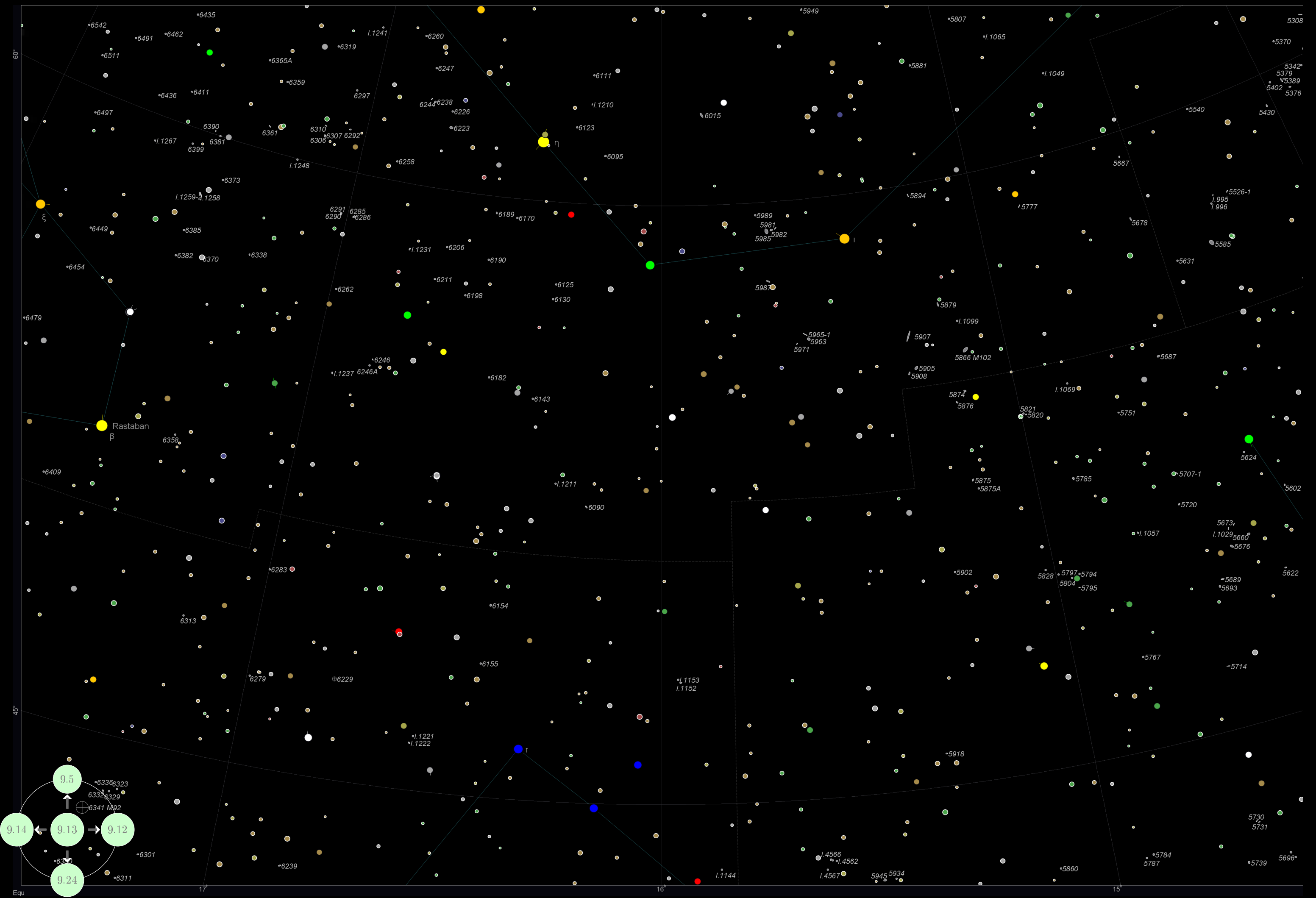
9.13 Mappa 13 25° attorno 16.0h, 54.0° (Draco)
